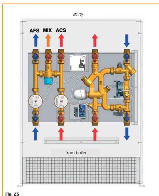
Fig. 23 Vertikální instalace se vstupy zespona
