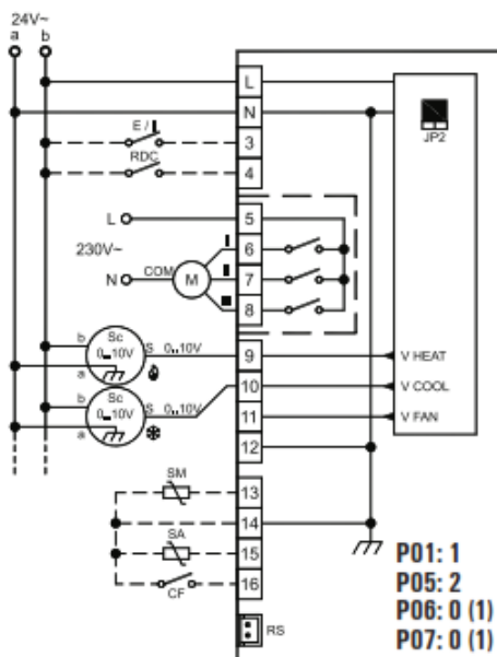
Obr. 10: Schéma zapojení pro 2 servopohony 0...10 V 24 V~ u 4trubkových systémů s jedním 230V třírýchlostním motorem.
